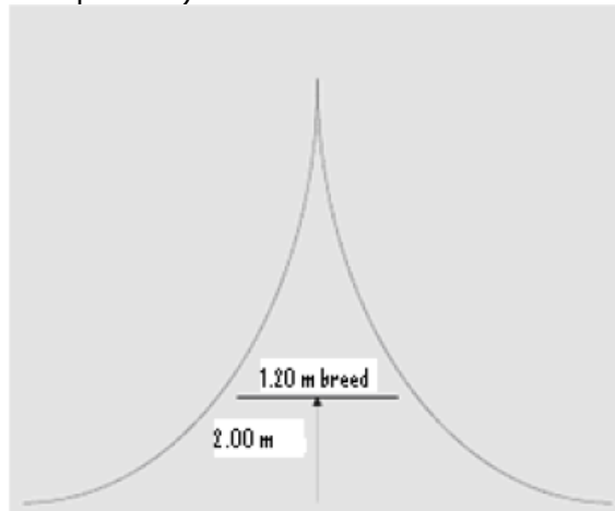
Meetpunt uitgangsbreedte tent (zijaanzicht)
